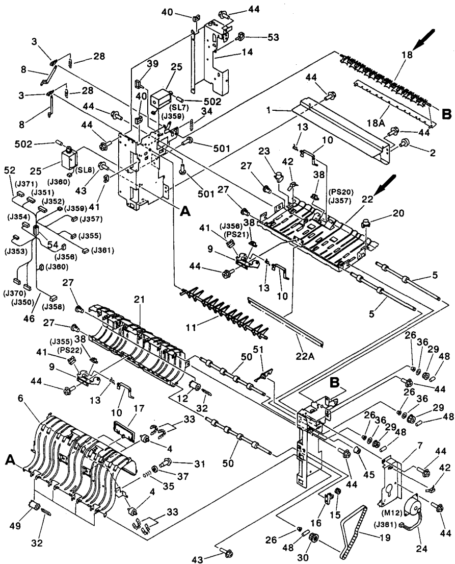
FIGURE Q30A FEEDER ASSEMBLY (GP40) 搬送部 (GP40)
