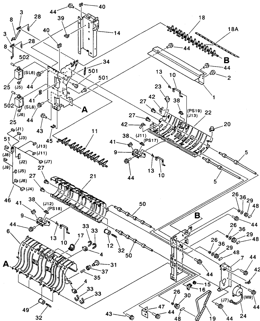
搬送部 (GP215)
